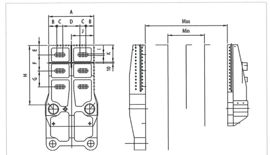
模板尺寸圖 | Mold Platen Dimensions
