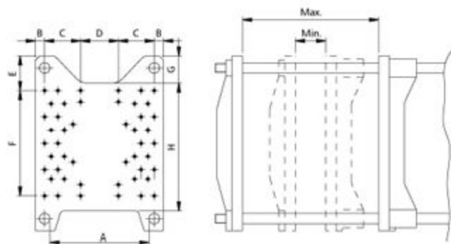
模板尺寸圖
